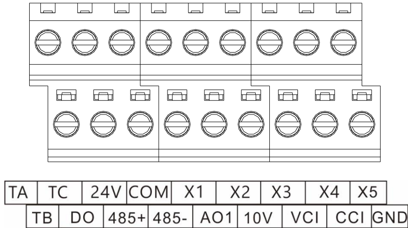
Рис. 3-5 Клеммы цепи управления (базовое исполнение)
