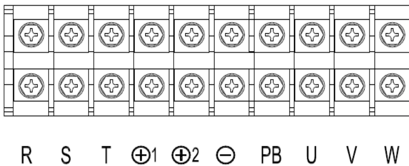
Рис. 3-4 Клеммы силовых цепей ПЧ мощностью 37 ... 630,0кВт
