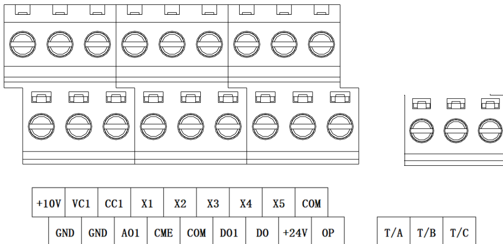
Рис. 3-6 Клеммы цепи управления (для ПЧ с опцией подключения платы расширения)
